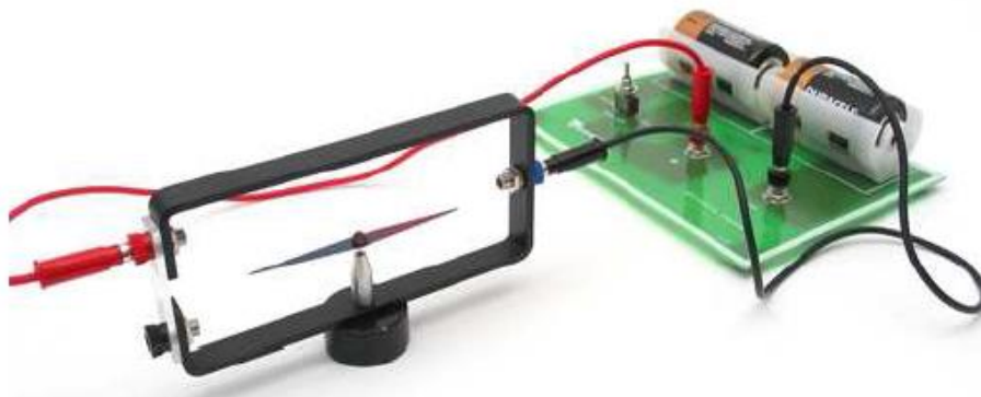
Figura 2. Aspecto final do experimento de Oersted (montado).
