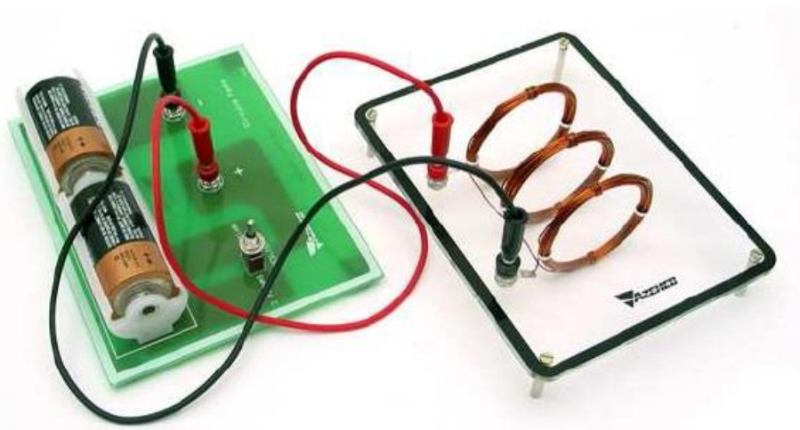
Figura 4. Aspecto final do experimento do solenoide (montado)
