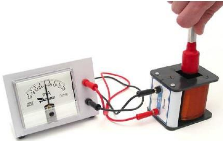
Figura 7. Aspecto final do experimento de indução eletromagnética (montado)
